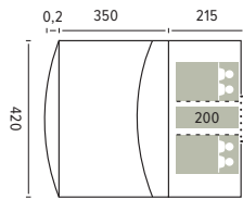
Dimensiones avance hinchable
