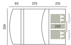
Dimensiones avance estructura de metal
