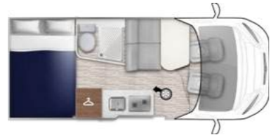
E-Van 2 →5990 mm
