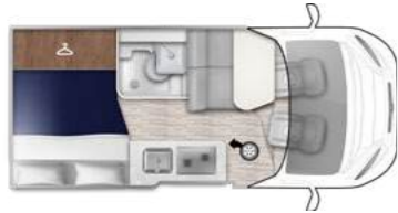
E-Van K2 →5410 mm
