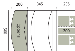
DIMENSIONES CON TOLDO CLÁSICO
